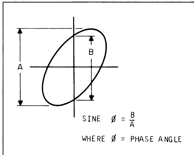
Fig. 41. Phase shift calculation.
